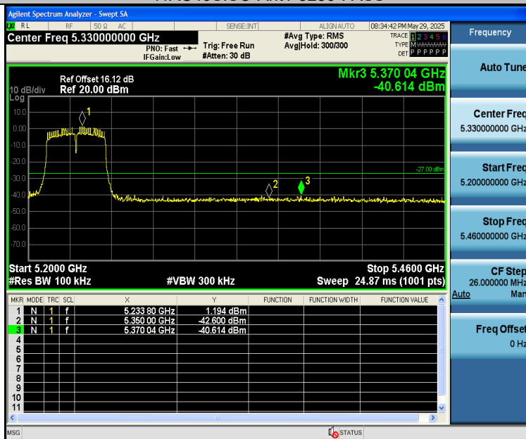
11AC80SISO-Ant1-5210-PASS
