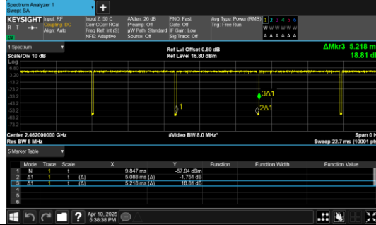
IEEE 802.11n_20MHz_Channel 11
