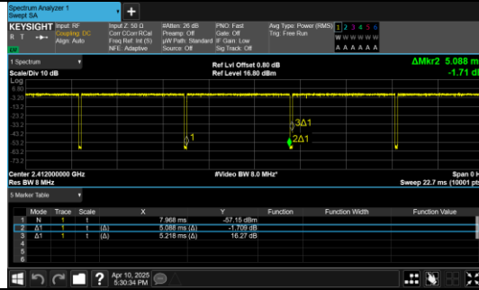
IEEE 802.11n_20MHz_Channel 1
