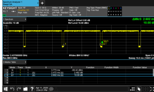
IEEE 802.11n_40MHz_Channel 6
