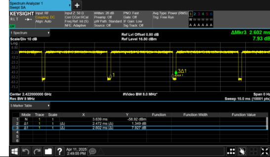
IEEE 802.11n_40MHz_Channel 3
