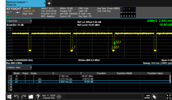
IEEE 802.11n_40MHz_Channel 9
