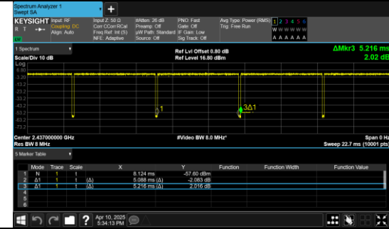
IEEE 802.11n_20MHz_Channel 6
