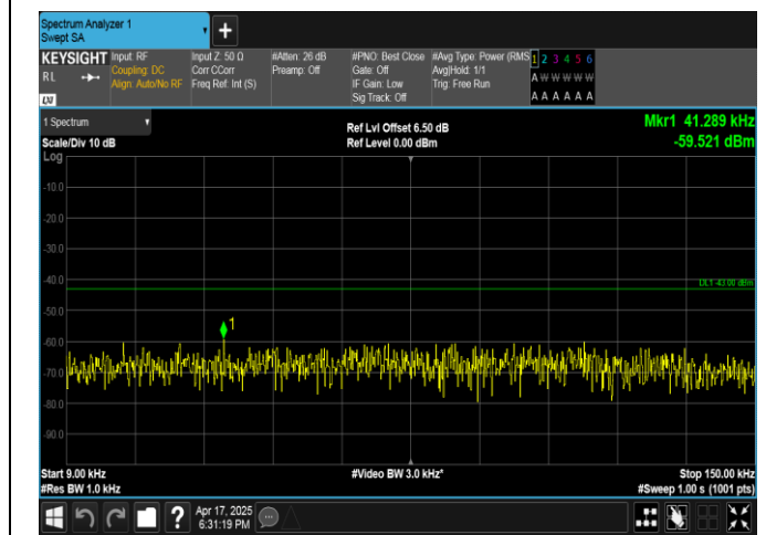
Band4-20MHz-QPSK-20175-1RB#0-0.009~0.15-PASS
