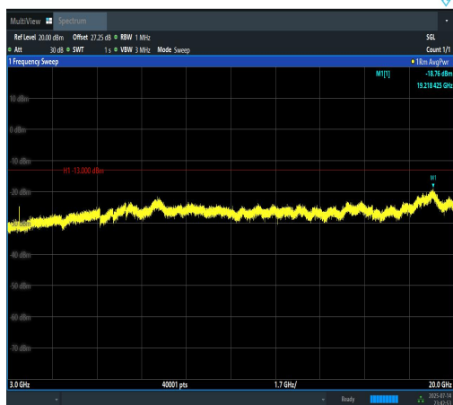
Band4-10MHz-QPSK-20000-50RB#0-3000~200 00-PASS
