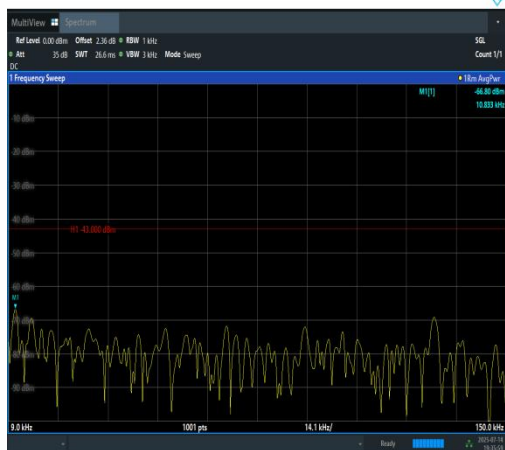
Band4-1.4MHz-QPSK-20393-6RB#0-0.009~0.15 -PASS
