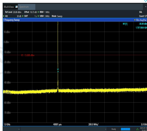
Band4-1.4MHz-QPSK-20393-6RB#0-1000~3000 -PASS
