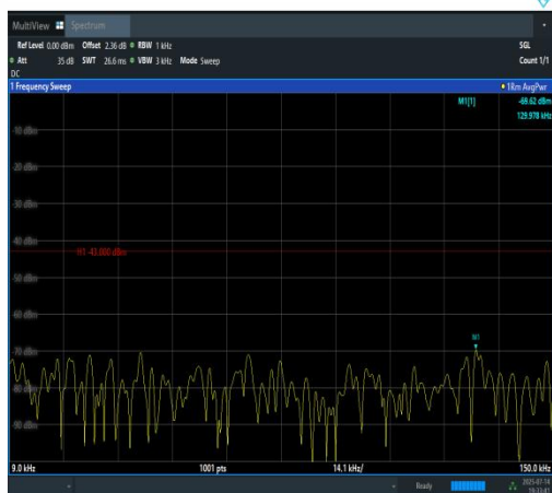
Band4-1.4MHz-QPSK-20393-1RB#0-0.009~0.15 -PASS
