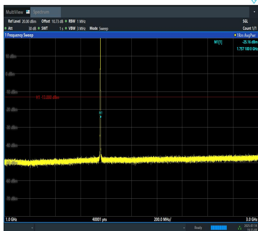
Band4-1.4MHz-QPSK-20393-1RB#5-1000~3000 -PASS
