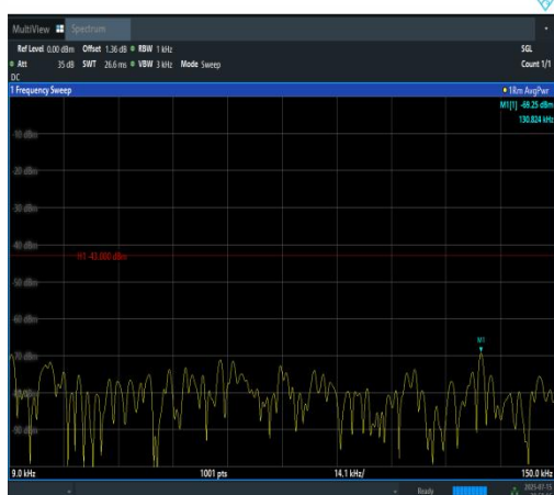
Band4-3MHz-QPSK-20175-1RB#0-0.009~0.15-P ASS
