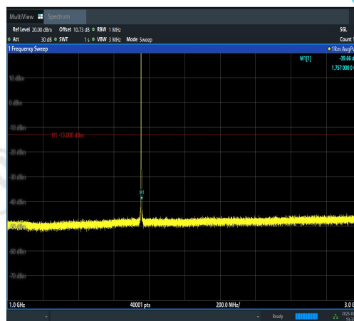
Band4-1.4MHz-QPSK-20393-1RB#0-1000~3000 -PASS
