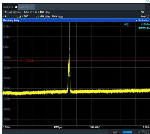
Band2-20MHz-QPSK-19100-1RB#99-1000~300 0-PASS
