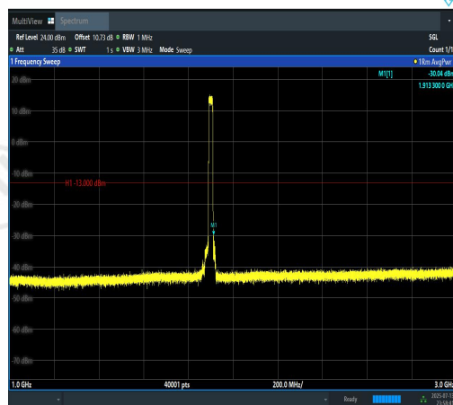
Band2-20MHz-QPSK-19100-100RB#0-1000~30 00-PASS 00-PASS
