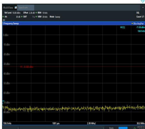
Band2-20MHz-QPSK-18900-1RB#99-0.15~30-P ASS
