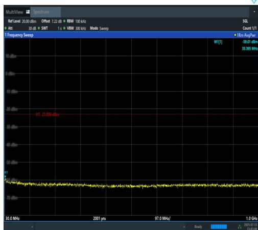
Band2-20MHz-QPSK-18900-1RB#0-30~1000-P ASS
