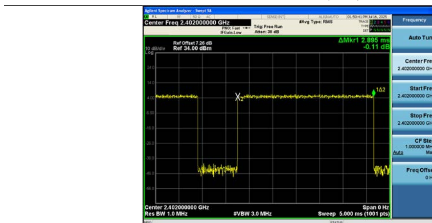
\pi/4 DQPSK : Dwell Time(Ch. 0)
