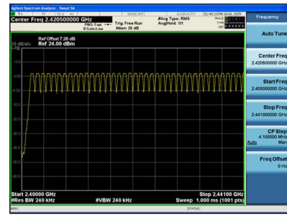
8DPSK (2.4 GHz - 2.441 GHz)
