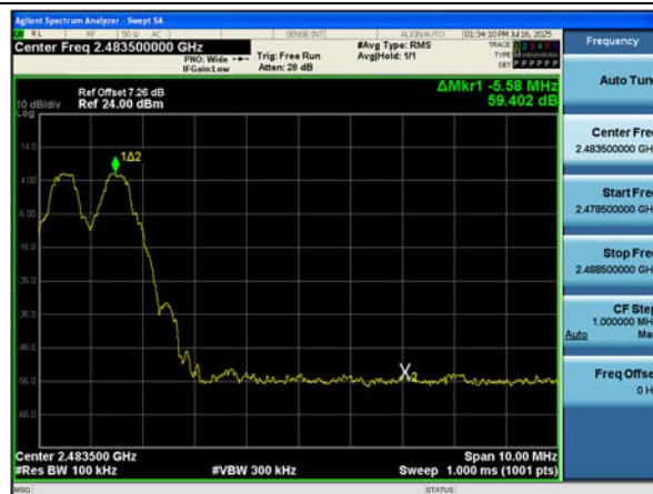
GFSK Band Edge(Ch. 78)
