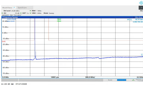
NTNV-n77(3700-3980)-PC1.5-30-20-L-DFT-QPSK-Inner_1RB_Left-3 000-6000-PASS
