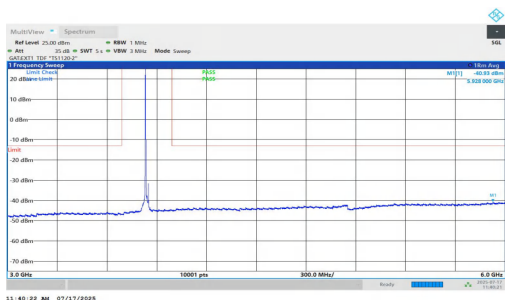
NTNV-n77(3700-3980)-PC1.5-30-20-M-DFT-QPSK-Inner_1RB_Left-3000-6000-PASS
