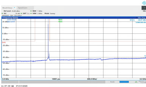
NTNV-n77(3700-3980)-PC1.5-30-20-H-DFT-QPSK-Inner_1RB_Left-3 000-6000-PASS
