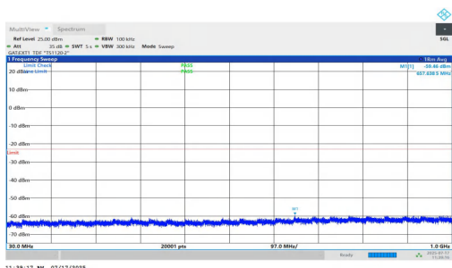
NTNV-n77(3700-3980)-PC1.5-30-20-M-DFT-QPSK-Inner_1RB_Left-30-1000-PASS
