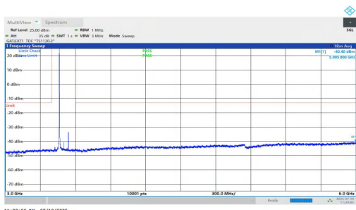
NTNV-n77(3450-3550)-PC1.5-30-80-M-DFT-QPSK-Inner_1RB_Left-3 000-6000-PASS
