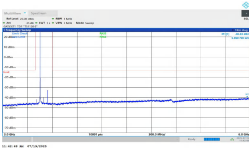
NTVN-n77(3450-3550)-PC1.5-30-90-L-DFT-QPSK-Inner_1RB_Left-3 000-6000-PASS
