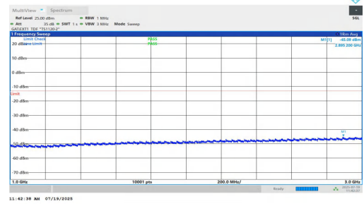
NTVN-n77(3450-3550)-PC1.5-30-90-L-DFT-QPSK-Inner_1RB_Left-10 00-3000-PASS
