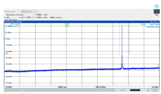
NTNV-n7-PC2-15-35-M-DFT-QPSK-Inner_1RB_Left-1000-3000-P ASS
