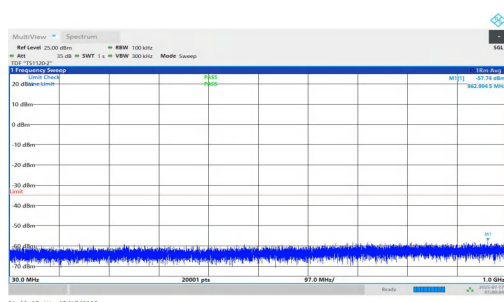
NTNV-n7-PC2-15-35-M-DFT-QPSK-Inner_1RB_Left-30-1000-PA SS
