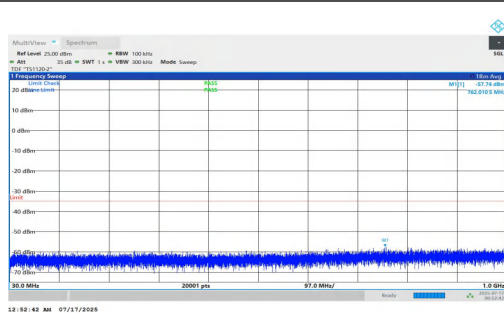
NTNV-n7-PC2-15-30-M-DFT-QPSK-Inner_1RB_Left-30-1000-PA SS
