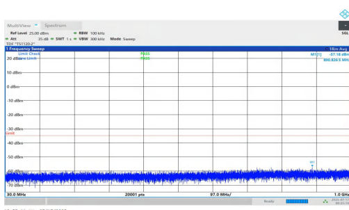
NTNV-n7-PC2-15-30-H-DFT-QPSK-Inner_1RB_Left-30-1000-P ASS
