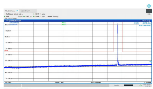
NTNV-n7-PC2-15-30-H-DFT-QPSK-Inner_1RB_Left-1000-3000-P ASS
