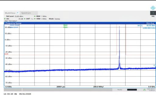
NTNV-n7-PC2-15-30-M-DFT-QPSK-Inner_1RB_Left-1000-3000-P ASS
