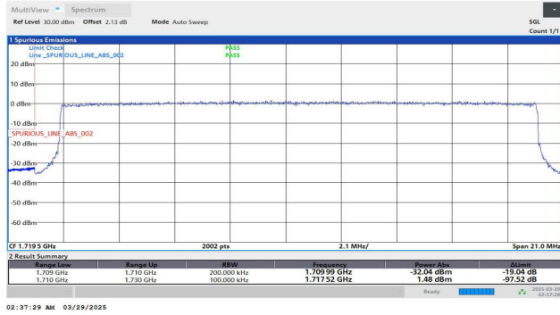
Band4-20MHz-QPSK-20050-100RB#0-PASS
