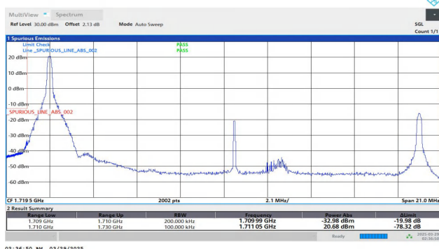
Band4-20MHz-QPSK-20050-1RB#0-PASS
