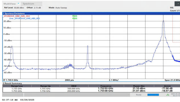
Band4-20MHz-QPSK-20300-1RB#99-PASS
