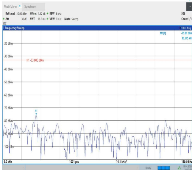
Band5-3MHz-QPSK-20635-1RB#0-0.009~0.15-PASS
