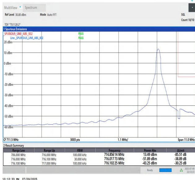
Band12_10MHz_QPSK_23130_1_High
