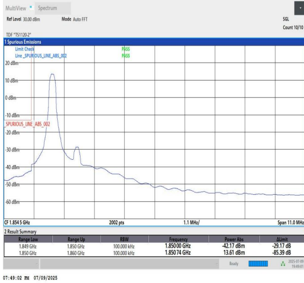
Band2_10MHz_QPSK_18650_1_Low
