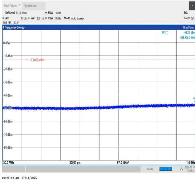
Band2-20MHz-QPSK-19100-PASS
