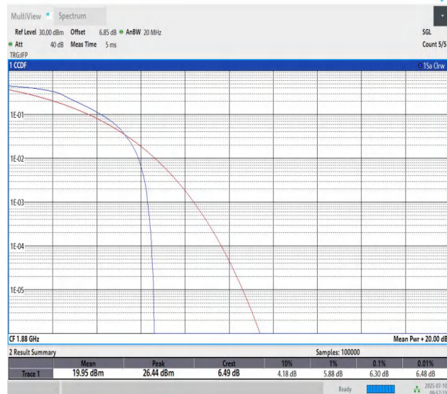
Band2-20MHz-QPSK-18900-PASS
