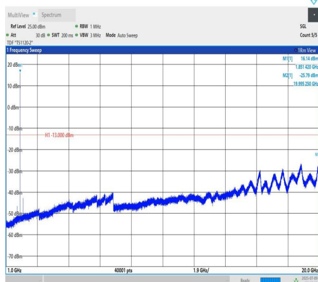
Band2-20MHz-QPSK-18700-PASS
