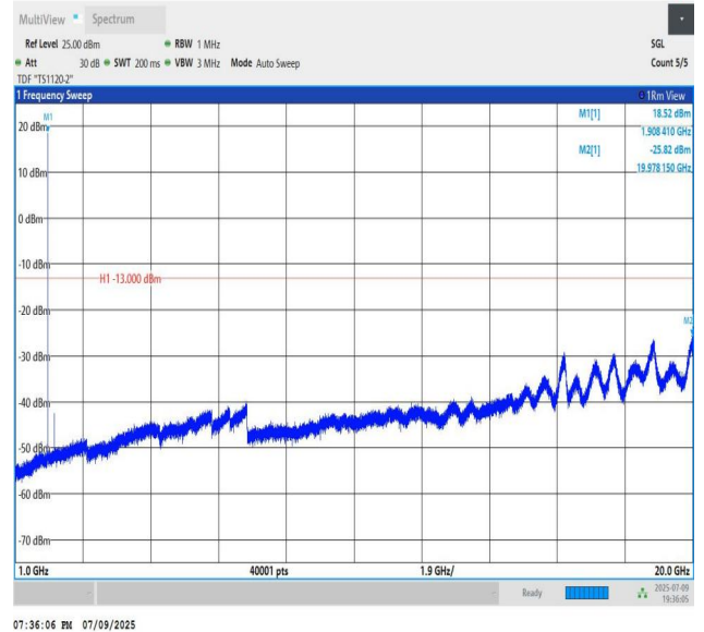
Band2-20MHz-QPSK-19100-PASS
