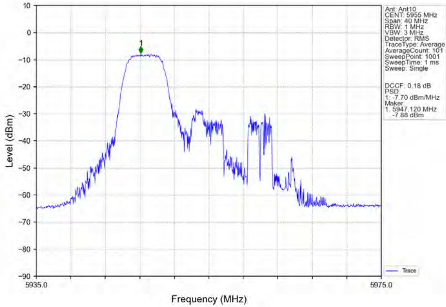
802.11ax(HEW20) LCH 5955MHz RU52 Left MIMO NTN
