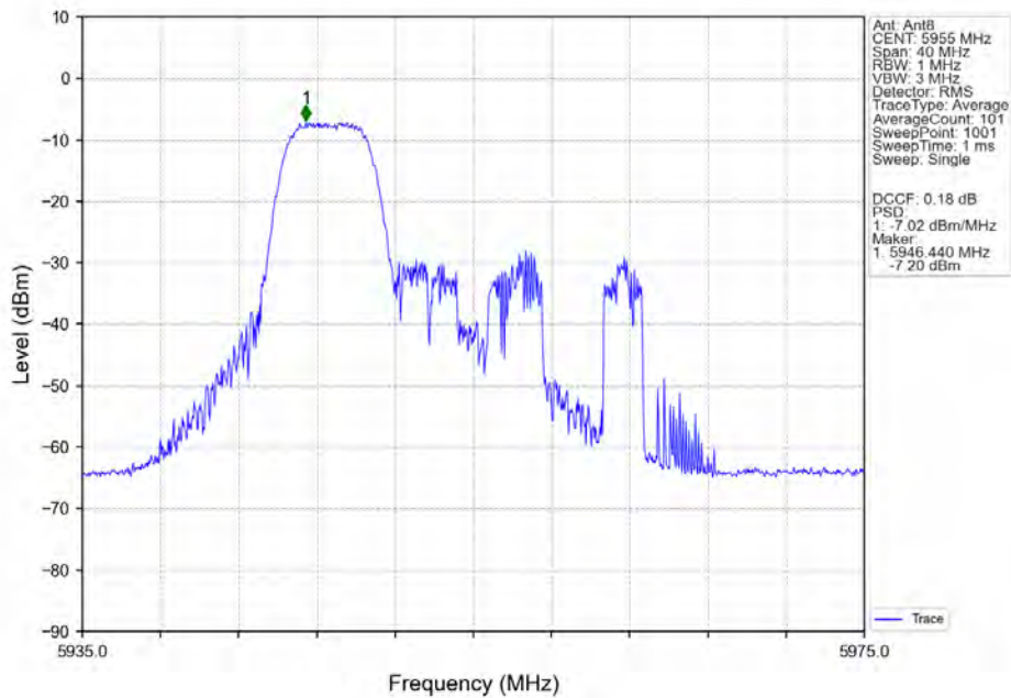
802.11ax(HEW20) LCH 5955MHz RU52 Left Ant8 NTN
