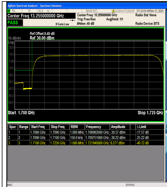
Band4_15MHz_QPSK_2025_75RB#0
