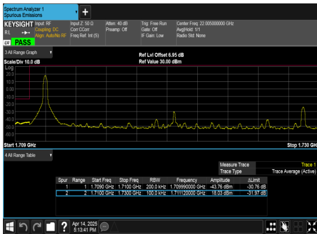
Band66-20MHz-QPSK-132072-1RB#0-PASS
