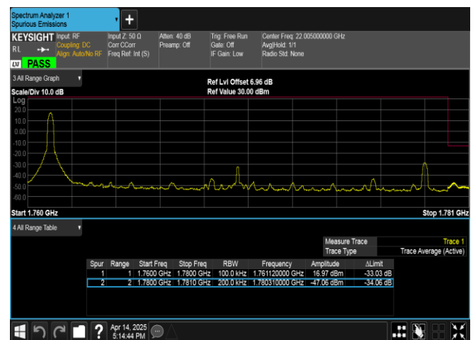
Band66-20MHz-QPSK-132572-1RB#0-PASS
