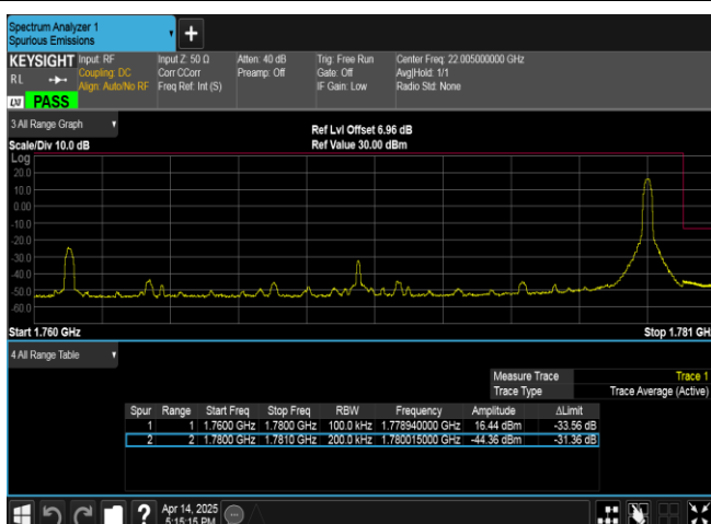
Band66-20MHz-QPSK-132572-1RB#99-PASS
