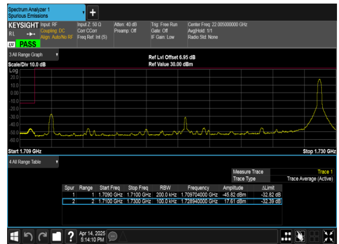
Band66-20MHz-QPSK-132072-1RB#99-PASS
