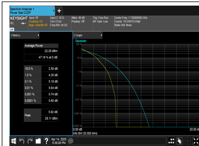
Band66-20MHz-QPSK-132072-1RB#0-PASS
