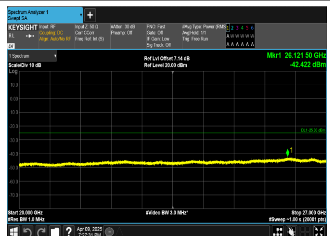
Band7-15MHz-16QAM-20825-1RB#0-20000~27000-PASS
