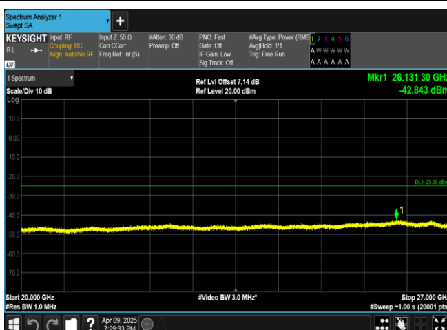
Band7-15MHz-16QAM-20825-1RB#74-20000~27000-PASS
