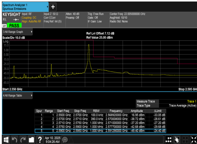
Band7-20MHz-QPSK-21350-1RB#99-PASS
