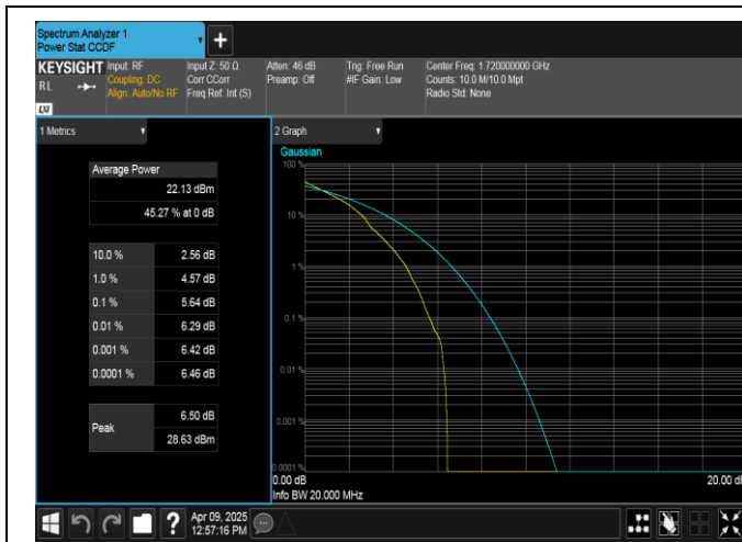
Band4-20MHz-QPSK-20050-1RB#0-PASS
