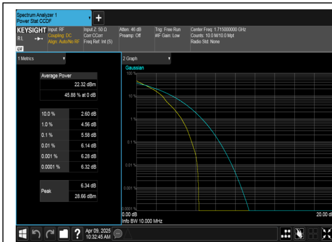
Band4-10MHz-QPSK-20000-1RB#0-PASS
