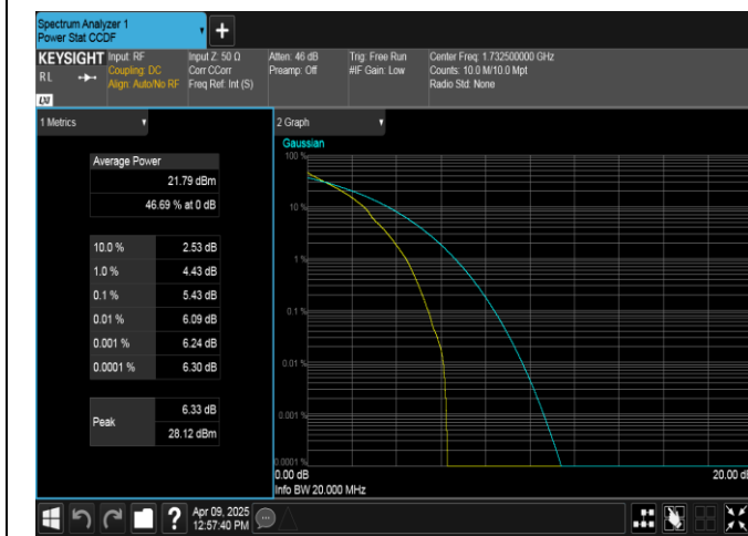
Band4-20MHz-QPSK-20175-1RB#0-PASS
