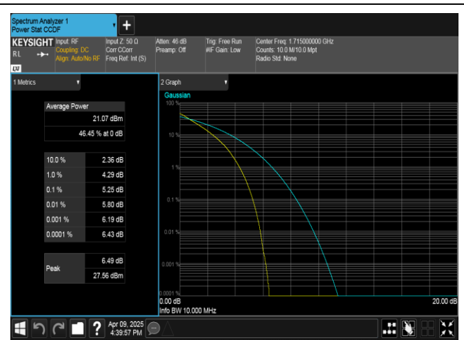
Band4-10MHz-QPSK-20000-50RB#0-PASS
