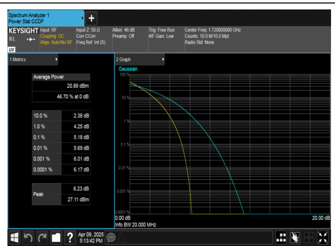
Band4-20MHz-QPSK-20050-100RB#0-PASS
