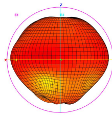
Total_3D_E1_5.85GHz
