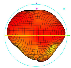
Total_3D_E2_5.85GHz
