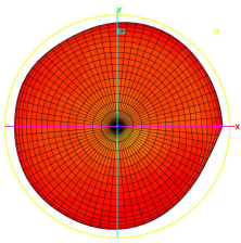
Total_3D_H_5.85GHz
