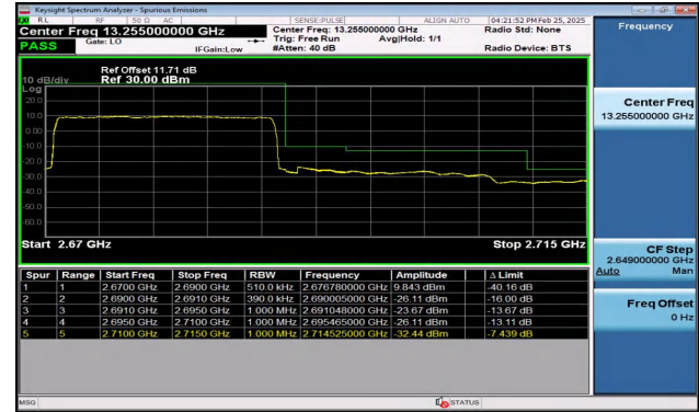
Band41_20MHz_QPSK_41490_100RB#0
