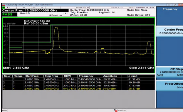
Band41_20MHz_QPSK_39750_1RB#0
