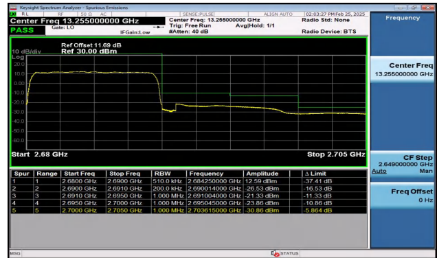
Band41_10MHz_QPSK_41540_50RB#0
