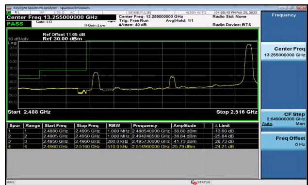
Band41_20MHz_QPSK_39750_1RB#99
