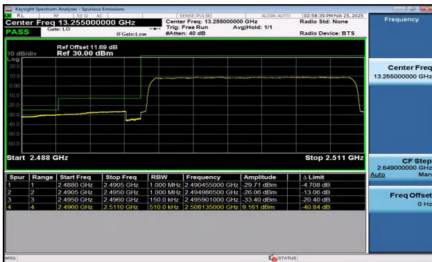
Band41_15MHz_QPSK_39725_75RB#0
