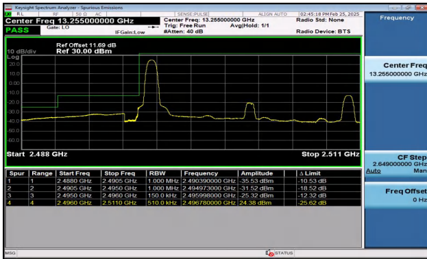
Band41_15MHz_QPSK_39725_1RB#0
