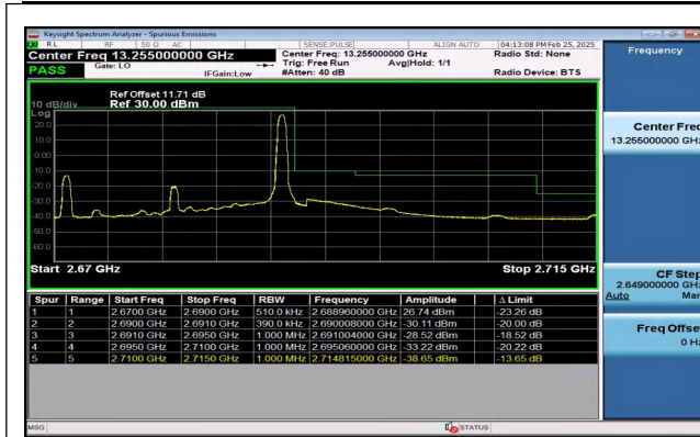
Band41_20MHz_QPSK_41490_1RB#99
