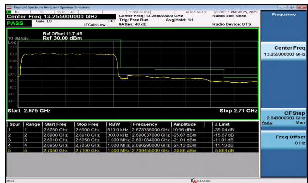
Band41_15MHz_QPSK_41515_75RB#0
