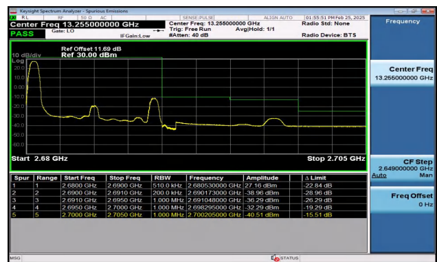
Band41_10MHz_QPSK_41540_1RB#0
