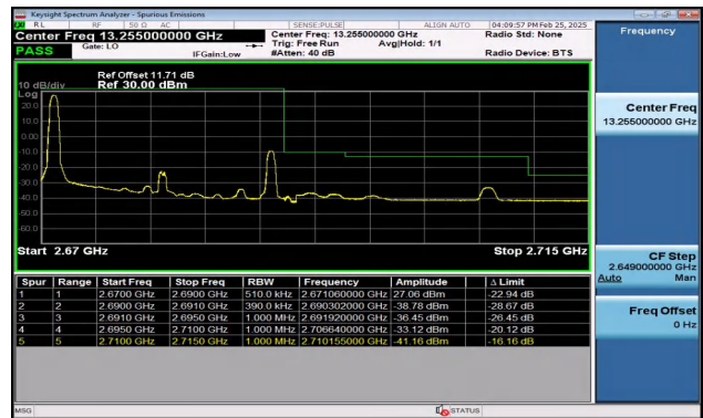
Band41_20MHz_QPSK_41490_1RB#0
