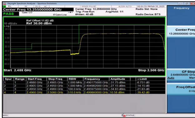
Band41_10MHz_QPSK_39700_50RB#0
