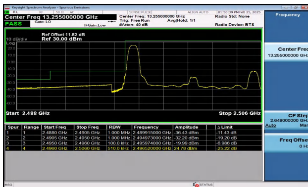
Band41_10MHz_QPSK_39700_1RB#0
