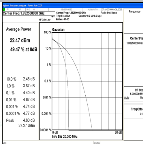
Band25-20MHz-QPSK-26365-1RB#0-PASS
