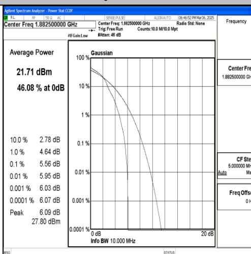
Band25-10MHz-16QAM-26365-1RB#0-PASS
