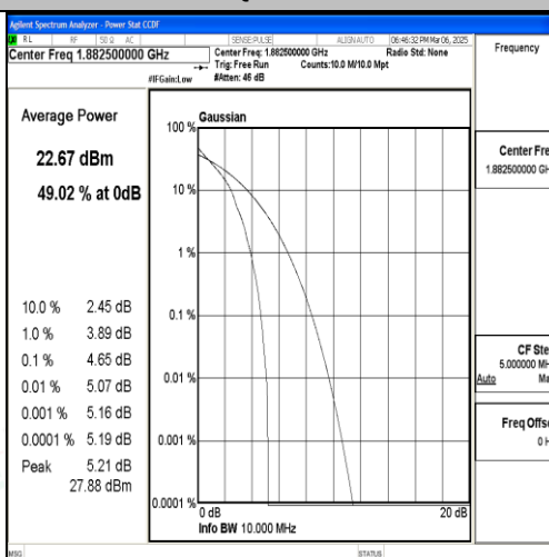
Band25-10MHz-QPSK-26365-1RB#0-PASS
