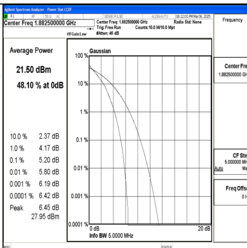
Band25-3MHz-QPSK-26365-15RB#0-PASS
