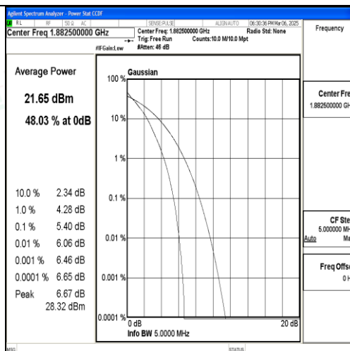
Band25-5MHz-QPSK-26365-25RB#0-PASS
