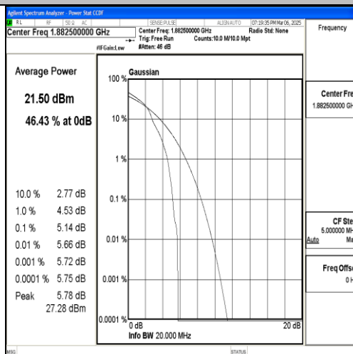
Band25-20MHz-16QAM-26365-1RB#0-PASS
