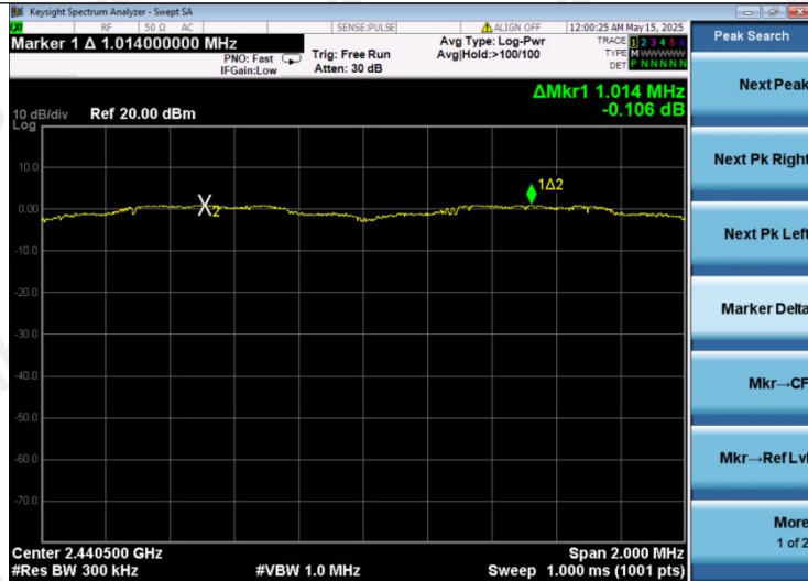
\pi/4 DQPSK
