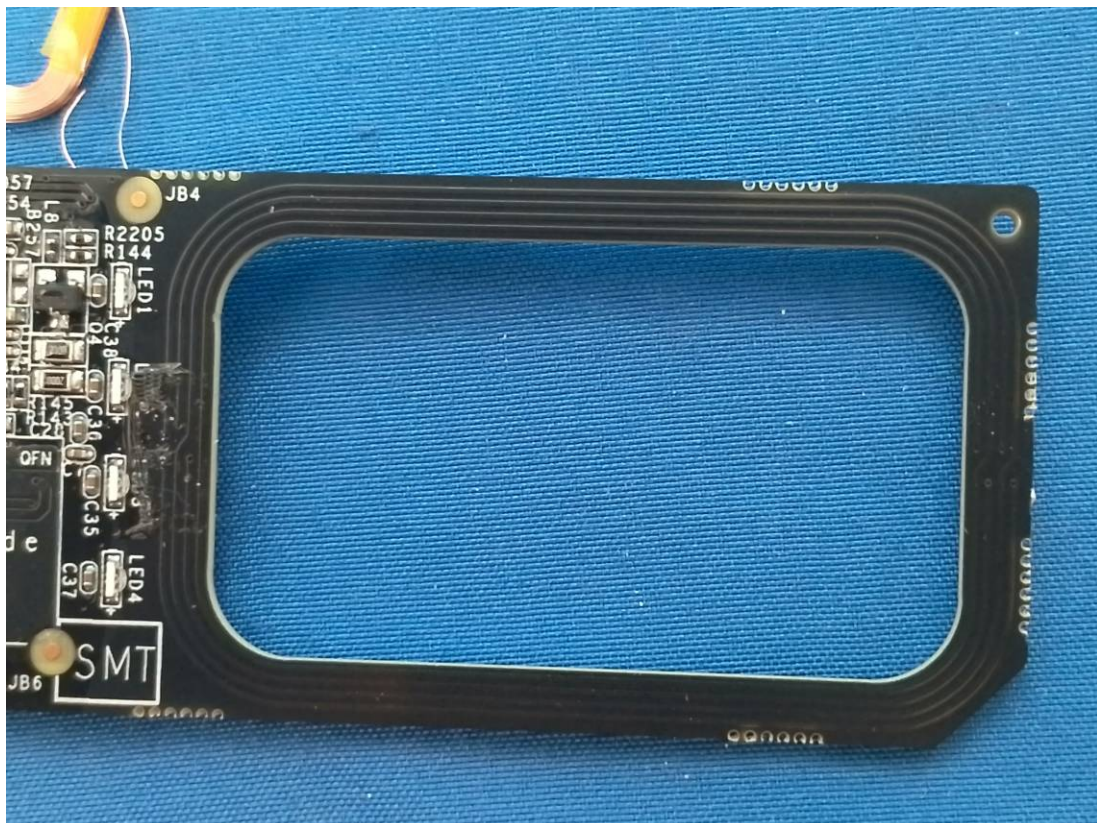
NFC 13.56MHz Antenna
