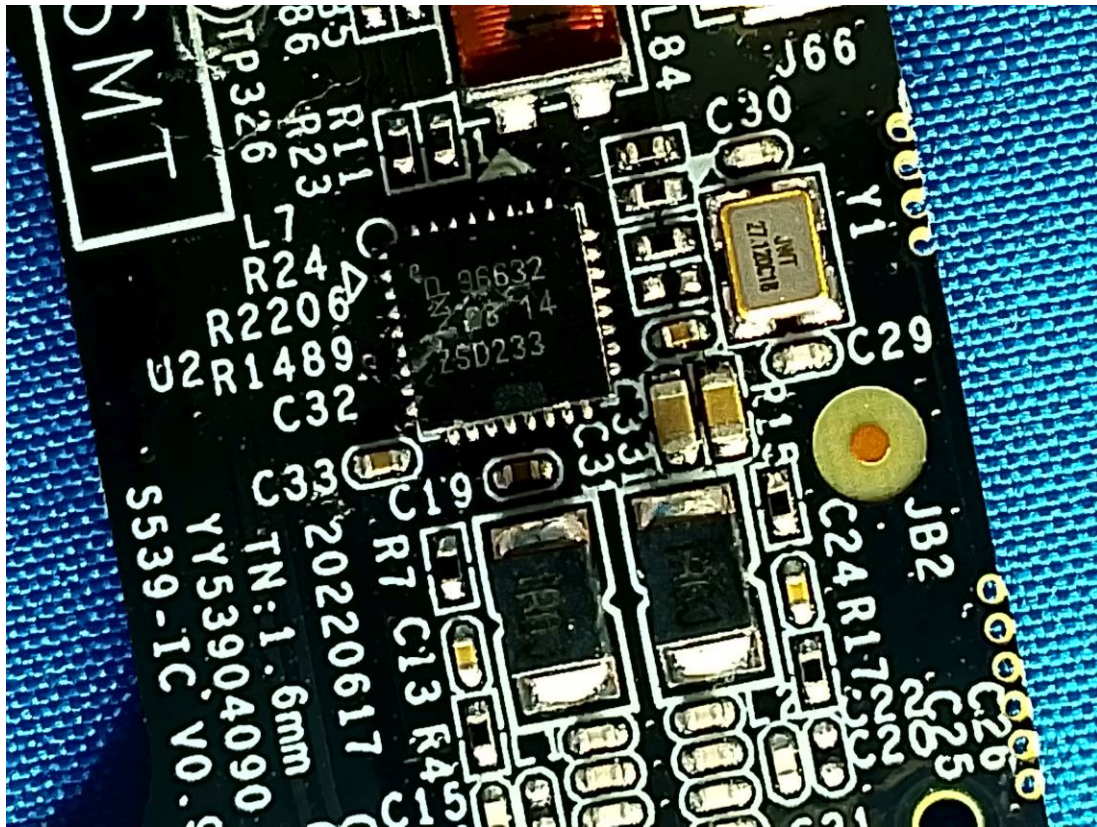
RFID 130.89kHz Antenna
