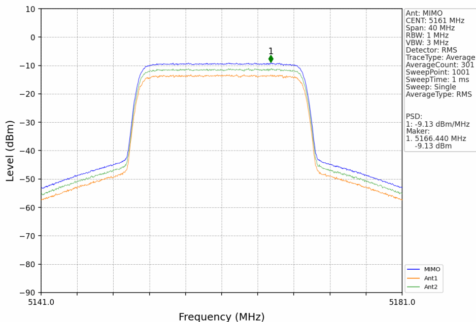
20M_LCH_5161MHz_MIMO_NTNV
