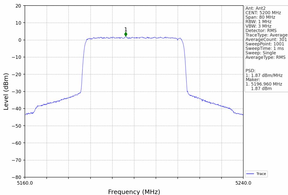
40M_MCH_5200MHz_MIMO_NTNV
