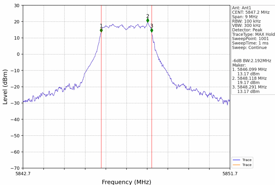
3M_HCH_5847.2MHz_Ant1_NTNV
