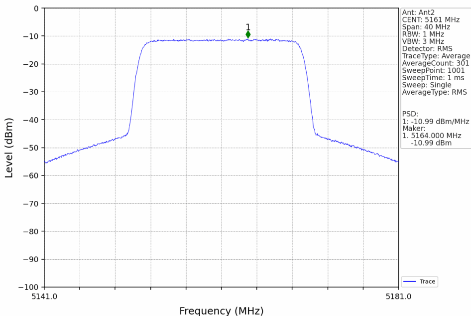
20M_LCH_5161MHz_MIMO_NTNV
