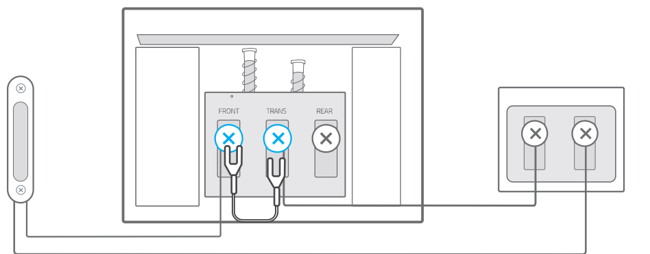
Pulsante del campanello esistente alla portad'ingresso.
