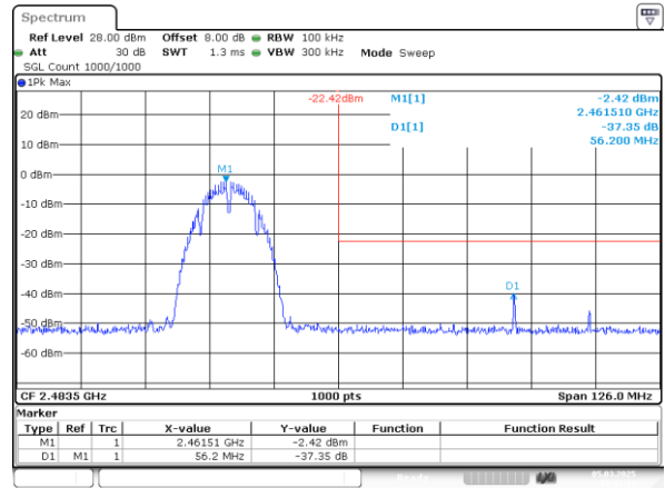
802.11b_2462MHz_Chain 0
