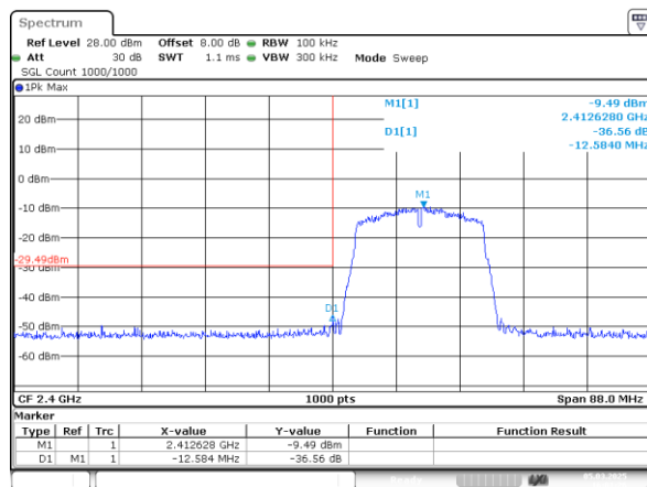
802.11n20_2412MHz_Chain 0
