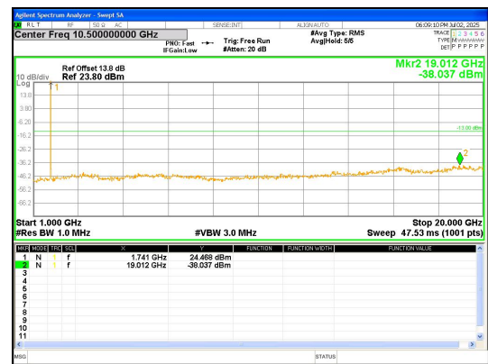
1000.0MHz-20000.0MHz Band 66 1.4MHz/1745.0/Mid QPSK 1@0
