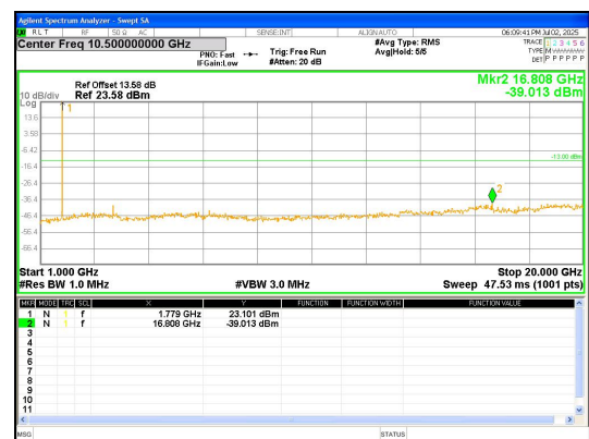
1000.0MHz-20000.0MHz Band 66 1.4MHz/1779.3/High QPSK 1@0
