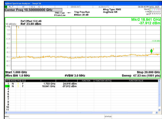
1000.0MHz-20000.0MHz Band 66 1.4MHz/1710.7/Low QPSK 1@0
