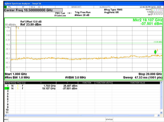
1000.0MHz-20000.0MHz Band 4 20MHz/1720.0/Low QPSK 1@0
