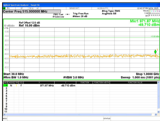
30.0MHz-1000.0MHz Band 4 20MHz/1732.5/Mid QPSK 1@0
