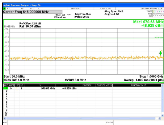
30.0MHz-1000.0MHz Band 4 10MHz/1732.5/Mid QPSK 1@0
