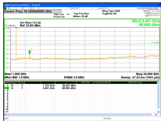
1000.0MHz-20000.0MHz Band 4 10MHz/1732.5/Mid QPSK 1@0
