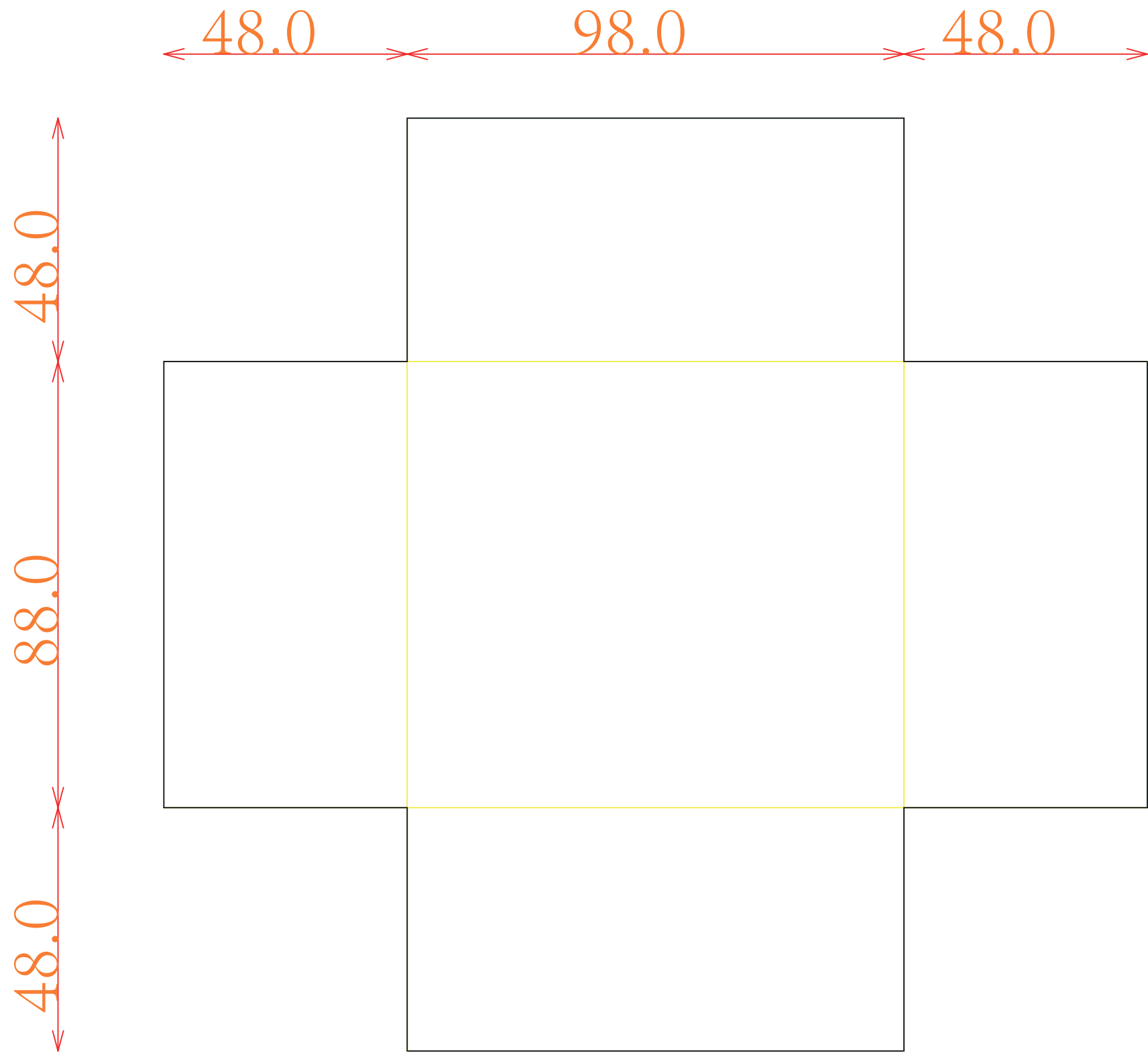
配件名称：地盒灰板 材料工艺：1200G单面白，V槽90度
