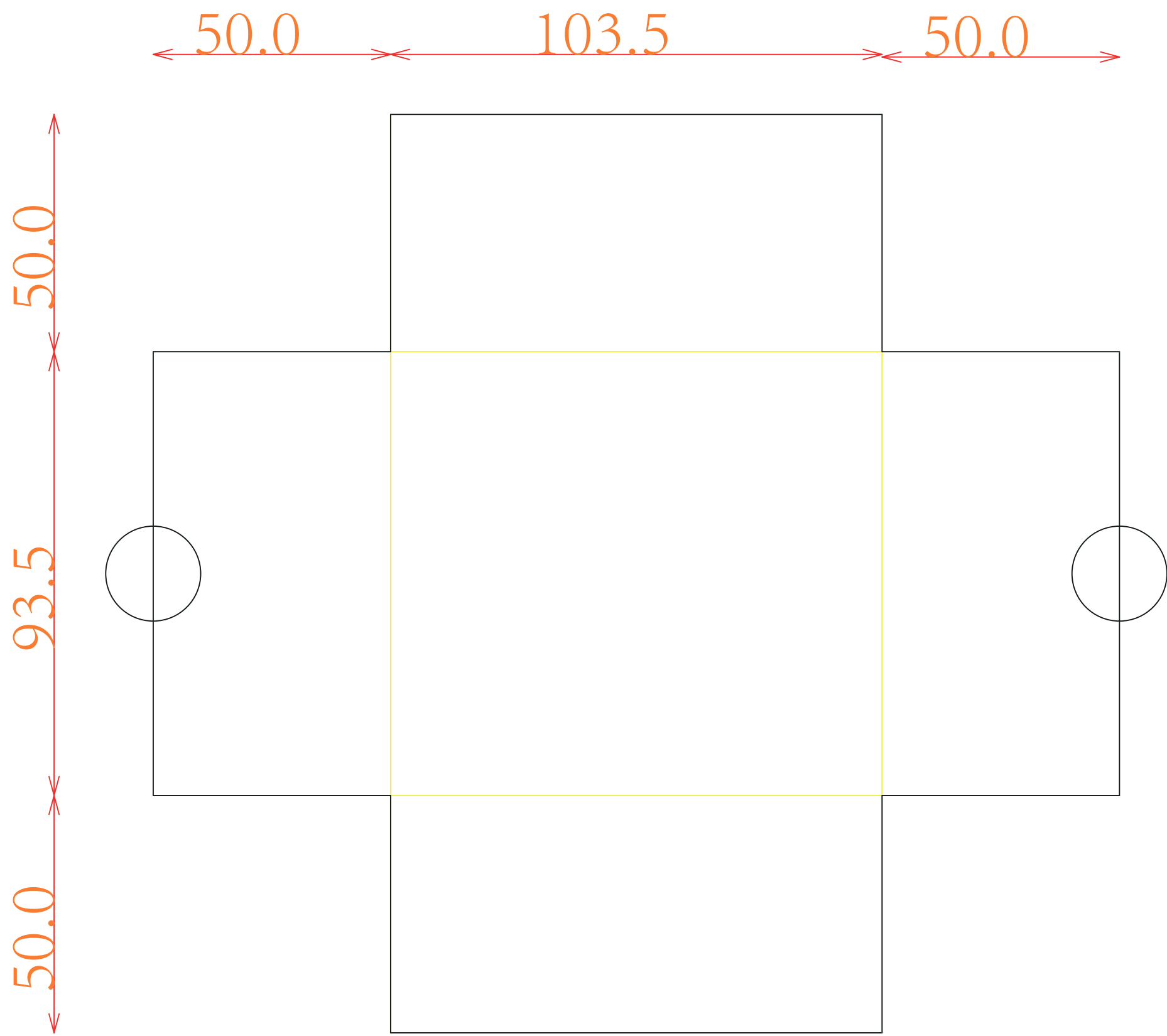
配件名称：天盖灰板 材料工艺：1200G单面白，V槽90度
