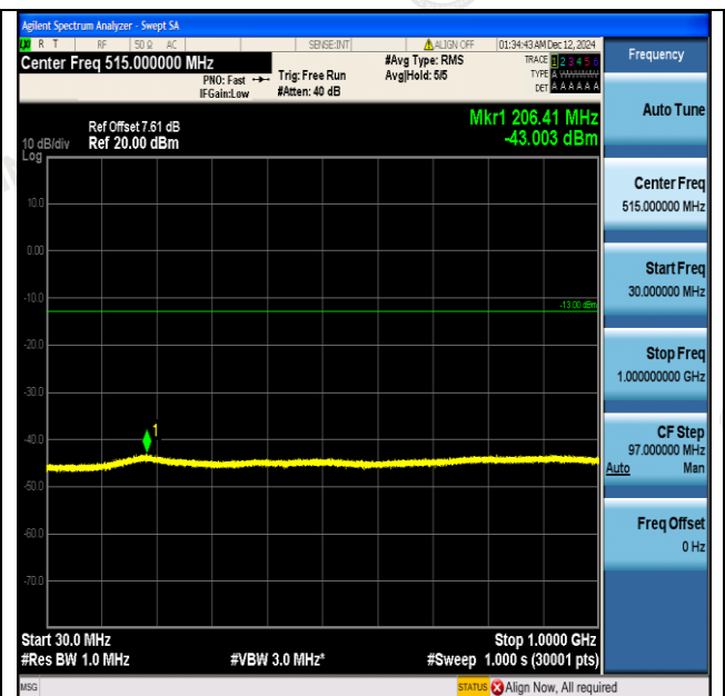
GPRS1900-810-0-30~1000MHz-PASS
