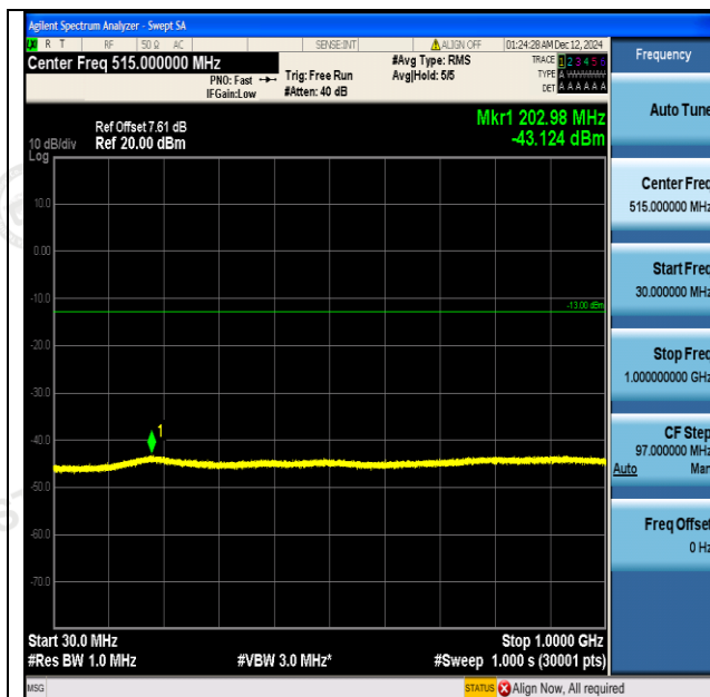
GSM1900-810-0-30~1000MHz-PASS
