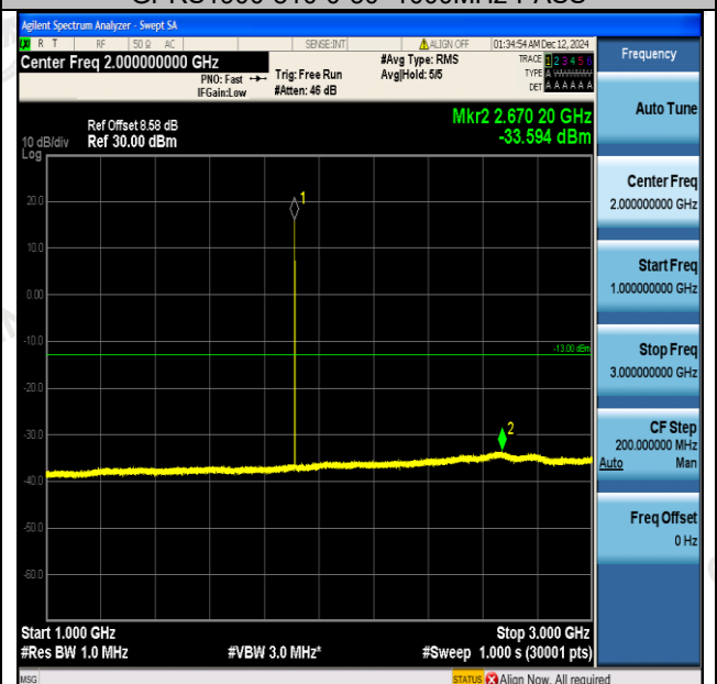
GPRS1900-810-0-1000~3000MHz-PASS
