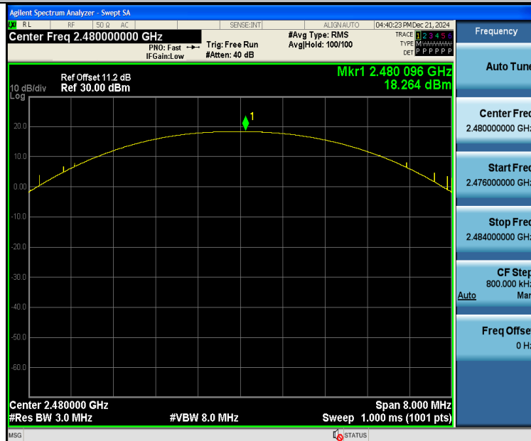
DH5-Ant4-2480-PASS
