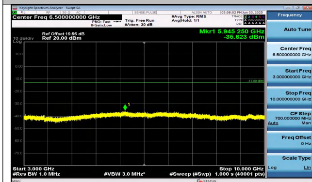
Band26(824-849)-10MHz-QPSK-26990-1RB#0-3000~100 00-PASS
