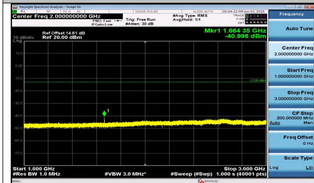
Band26(824-849)-10MHz-QPSK-26915-1RB#0-1000~300 0-PASS
