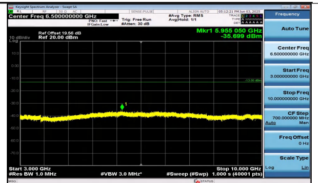
Band26(824-849)-10MHz-QPSK-26915-50RB#0-3000~10 000-PASS
