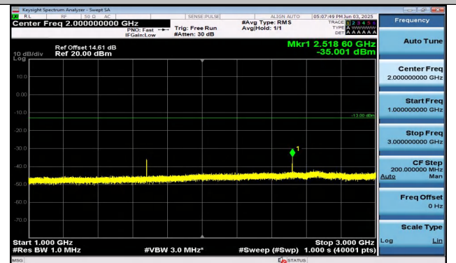
Band26(824-849)-10MHz-QPSK-26990-1RB#0-1000~300 0-PASS
