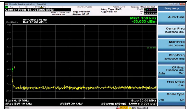
Band26(824-849)-10MHz-QPSK-26990-1RB#0-0.15~30-P ASS
