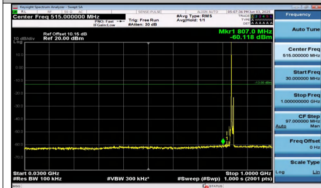
Band26(824-849)-10MHz-QPSK-26990-1RB#0-30~1000-P ASS
