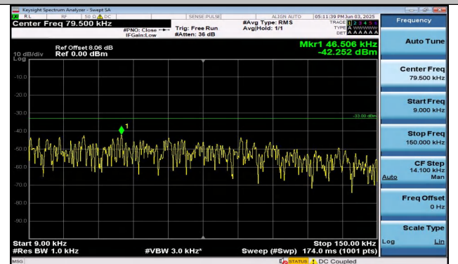
Band26(824-849)-10MHz-QPSK-26915-50RB#0-0.009~0.15- 15-PASS
