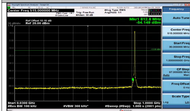
Band26(824-849)-3MHz-QPSK-26805-15RB#0-30~1000-P ASS
