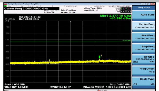
Band26(824-849)-3MHz-QPSK-26805-15RB#0-1000~300 0-PASS
