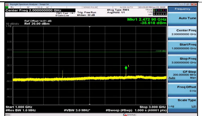
Band26(824-849)-3MHz-QPSK-26805-1RB#0-1000~3000-
