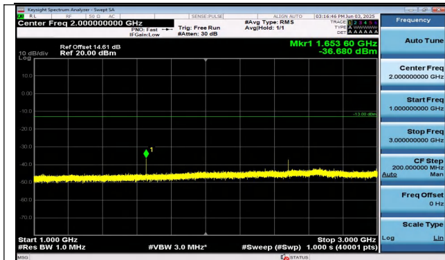
Band26(824-849)-3MHz-QPSK-26805-1RB#14-1000~300 0-PASS
