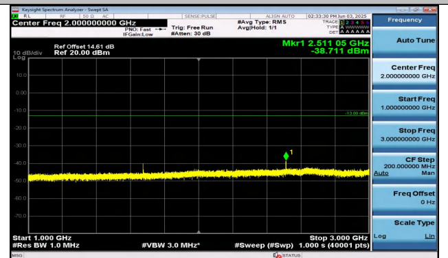
Band26(824-849)-1.4MHz-16QAM-26915-1RB#5-1000~3000-. 00-PASS
