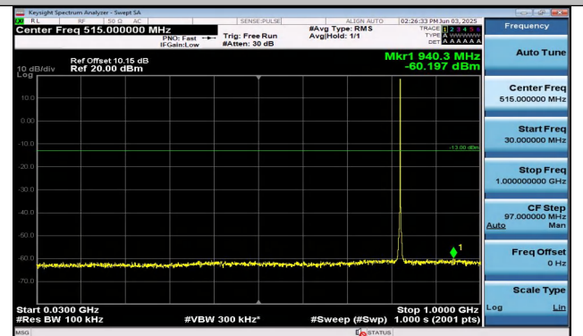
Band26(824-849)-1.4MHz-16QAM-26797-1RB#0-30~1000 -PASS
