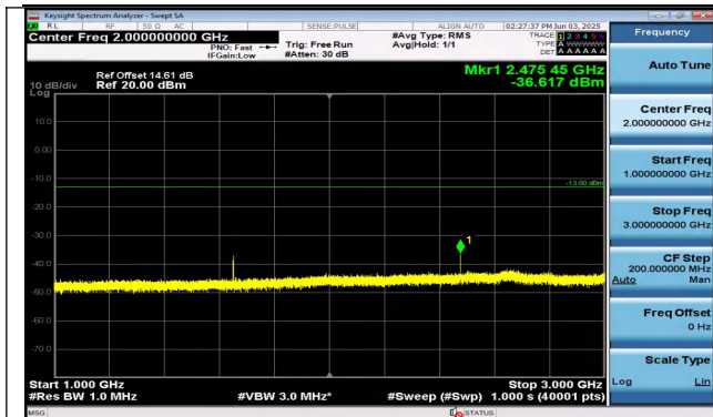
Band26(824-849)-1.4MHz-QPSK-26797-1RB#5-1000~300 0-PASS
