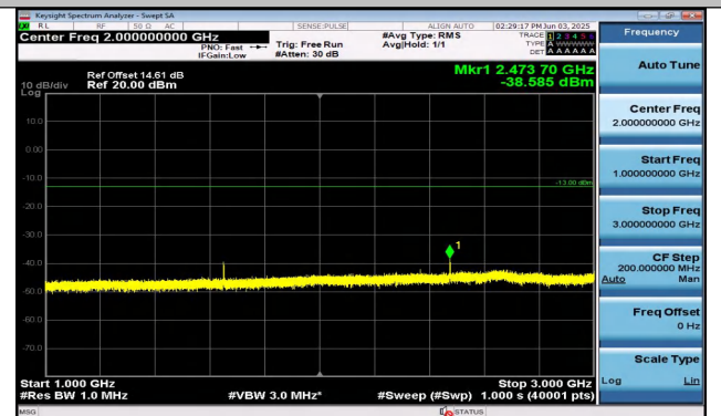
Band26(824-849)-1.4MHz-QPSK-26797-6RB#0-1000~300 0-PASS
