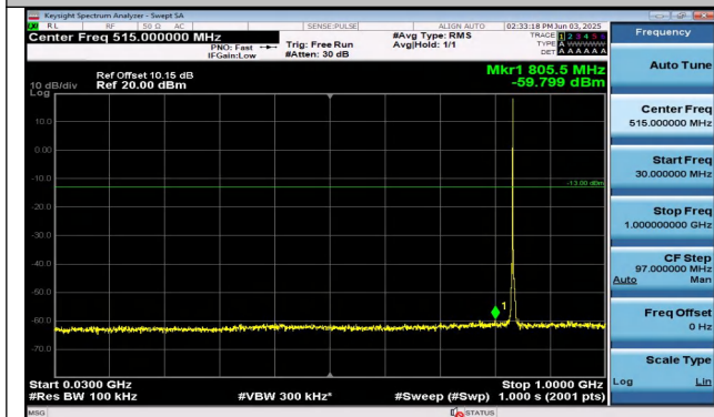
Band26(824-849)-1.4MHz-16QAM-26915-1RB#5-30~1000-. -PASS
