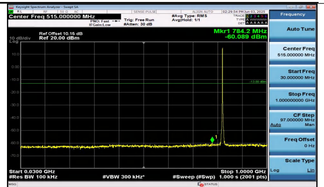
Band26(824-849)-1.4MHz-16QAM-26797-6RB#0-30~1000 -PASS
