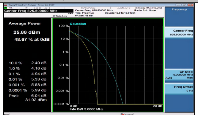
Band26(824-849)-3MHz-QPSK-26805-15RB#0-PASS
