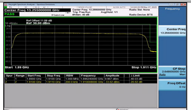
Band2-20MHz-QPSK-19100-1RB#99-PASS
