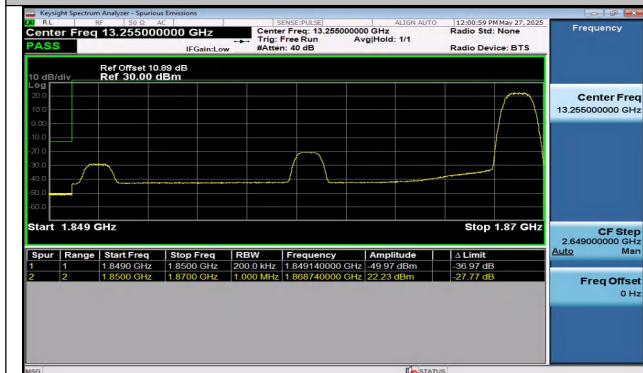
Band2-20MHz-16QAM-18700-1RB#0-PASS
