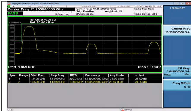
Band2-20MHz-QPSK-18700-1RB#0-PASS
