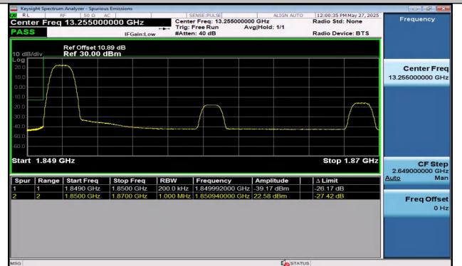
Band2-20MHz-QPSK-18700-1RB#99-PASS
