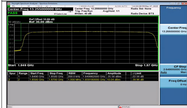
Band2-20MHz-QPSK-18700-100RB#0-PASS
