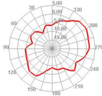
5160.000MHz H
