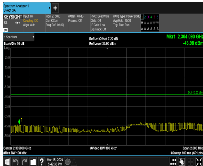
Band40-5MHz-QPSK-38725-25RB#0
