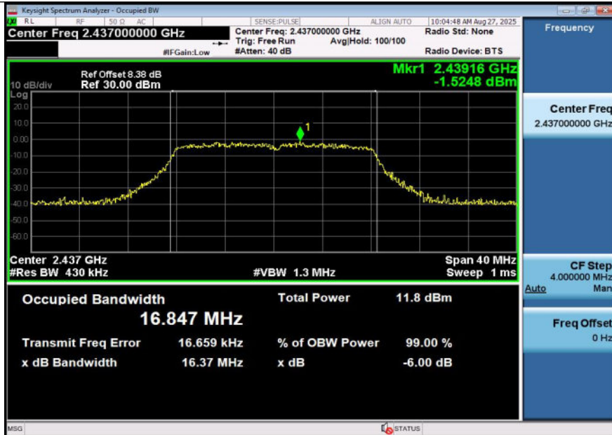
11G-Ant1-2437
