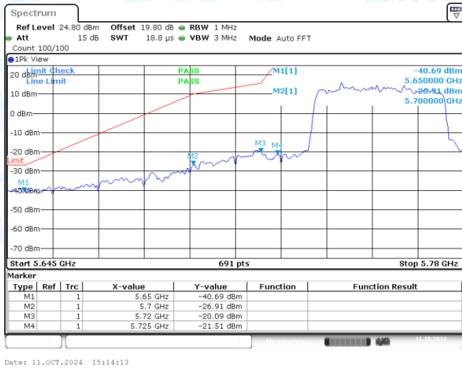
11AX40MIMO-Ant1-5755-PASS
