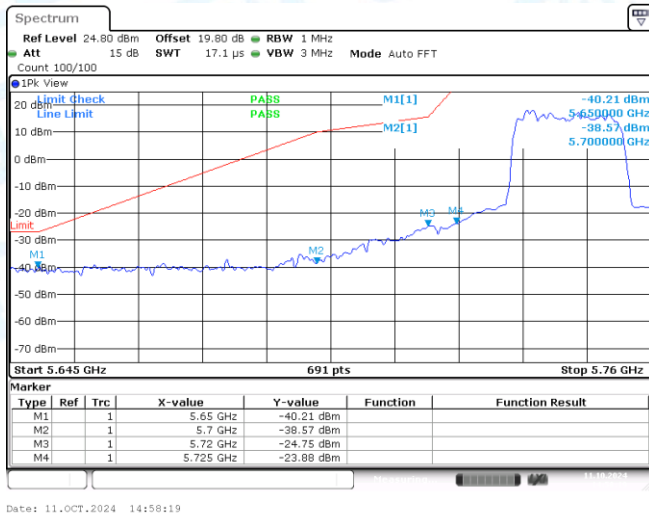
11AX20MIMO-Ant1-5745-PASS
