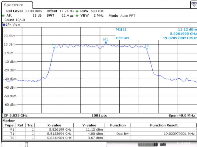
11AX20MIMO-Ant1-5825
