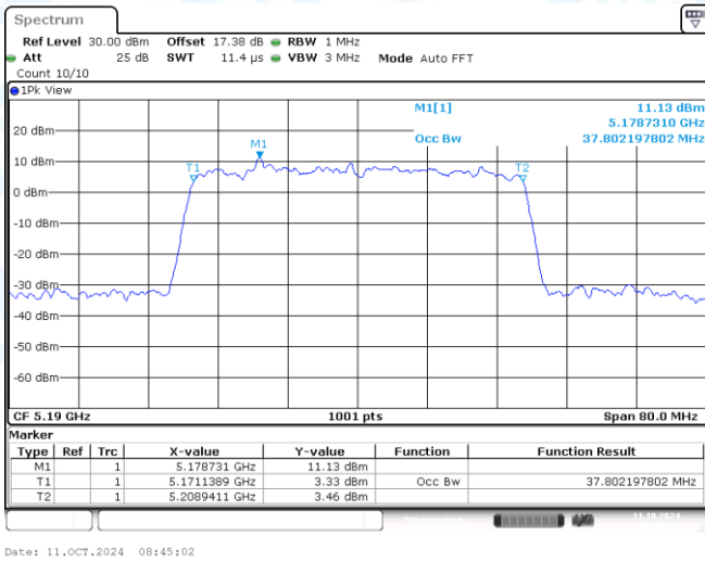
11AX40MIMO-Ant1-5190
