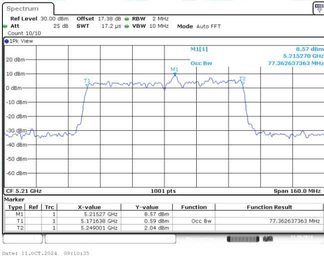
11AX80MIMO-Ant1-5210
