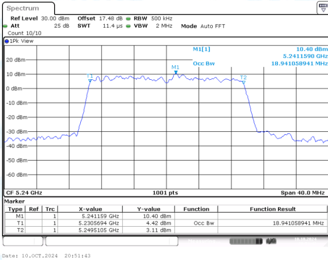
11AX20MIMO-Ant1-5240
