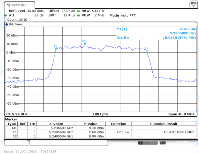
11AX20MIMO-Ant2-5240
