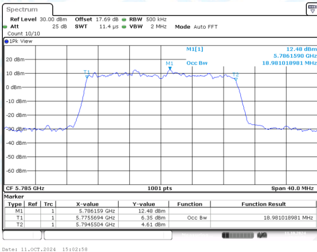
11AX20MIMO-Ant1-5785
