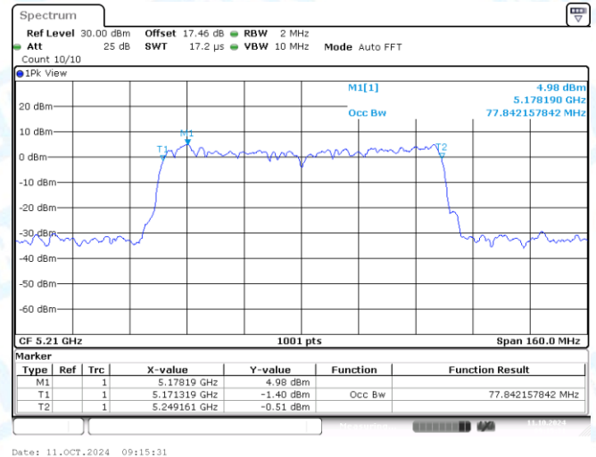
11AX80MIMO-Ant2-5210
