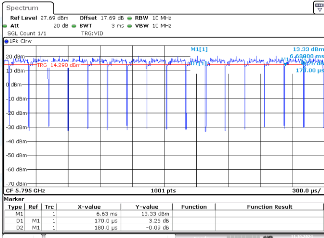
NTNV-11N40MIMO-Ant1-5795
