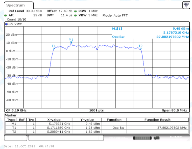
11AX40MIMO-Ant2-5190
