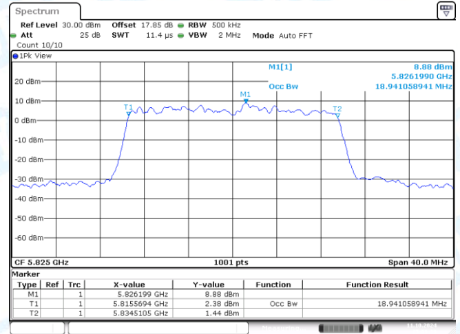
11AX20MIMO-Ant2-5825
