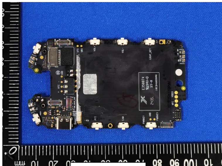
WWAN mani Antenna
