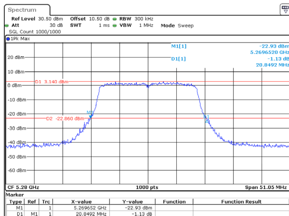
802.11ac20_5280MHz_Chain 0
