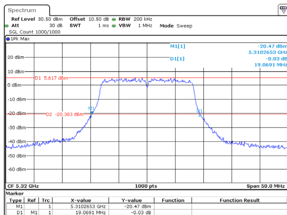
802.11a_5320MHz_Chain 2
