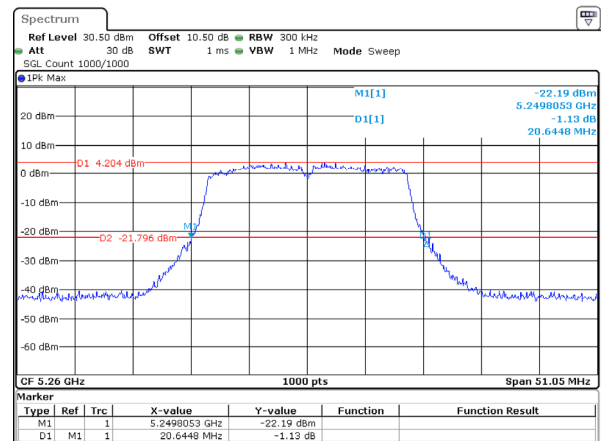
802.11ac20_5260MHz_Chain 3
