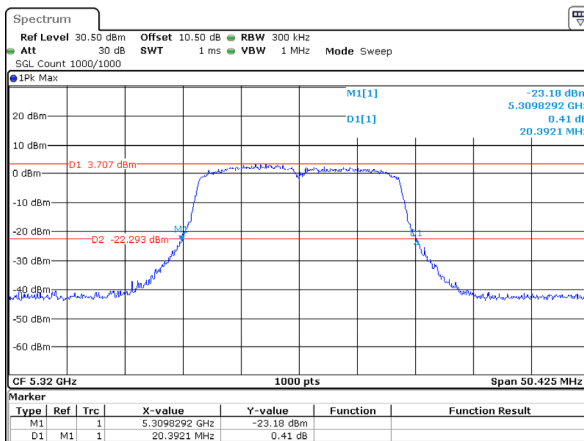
802.11ac20_5320MHz_Chain 2
