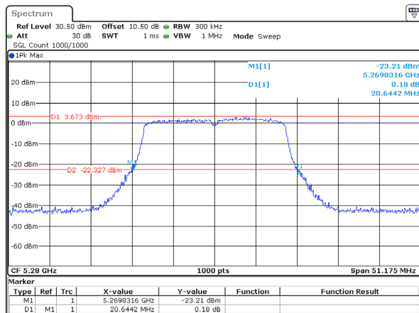
802.11ac20_5280MHz_Chain 1
