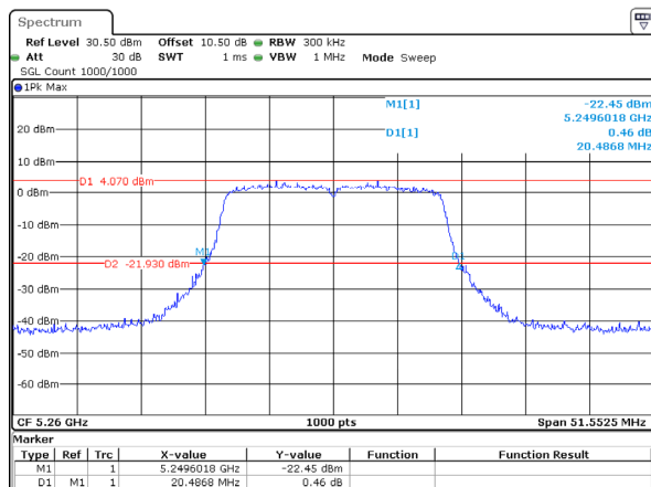
802.11ac20_5260MHz_Chain 0
