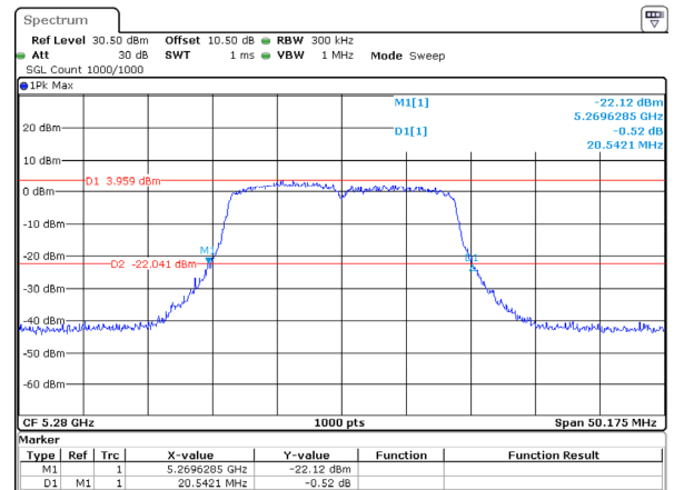
802.11ac20_5280MHz_Chain 2
