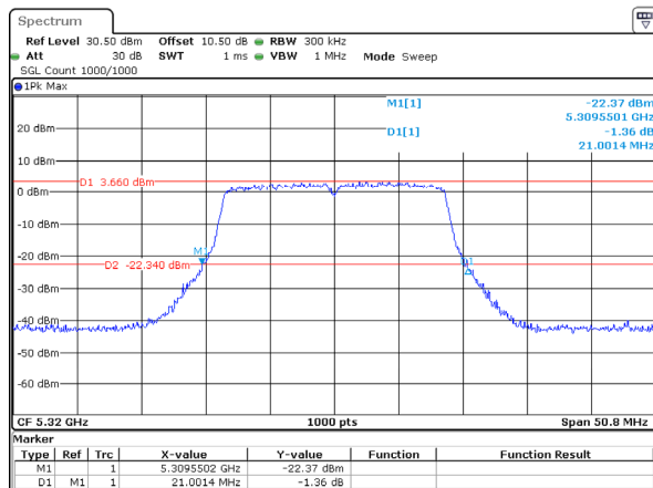
802.11ac20_5320MHz_Chain 1
