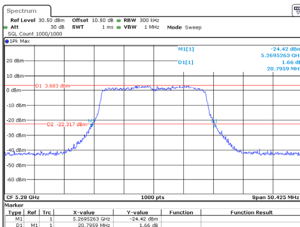
802.11ac20_5280MHz_Chain 3
