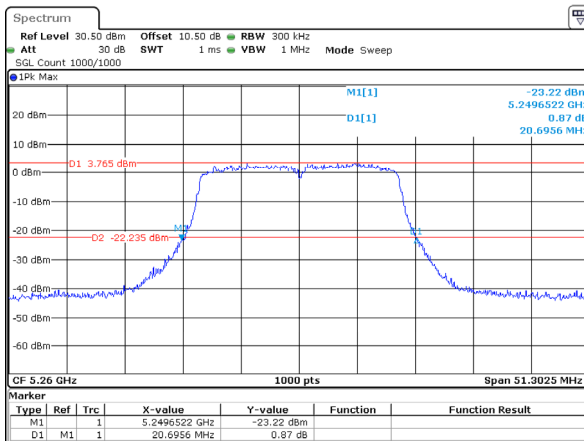
802.11ac20_5260MHz_Chain 2
