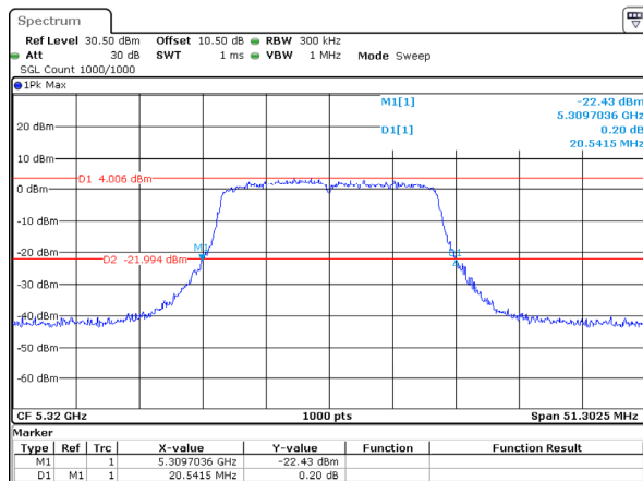
802.11ac20_5320MHz_Chain 0
