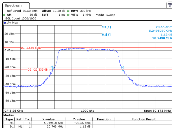
802.11ac20_5260MHz_Chain 1
