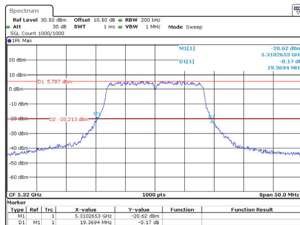
802.11a_5320MHz_Chain 3
