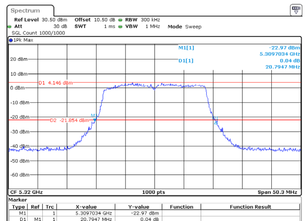
802.11ac20_5320MHz_Chain 3
