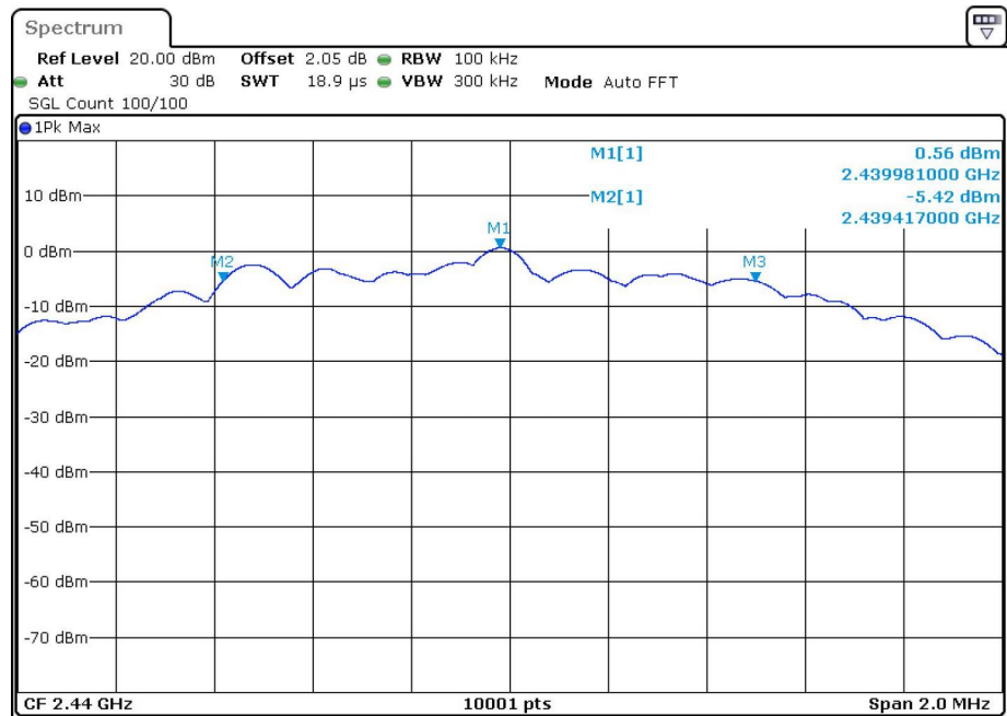
-6dB Bandwidth BLE 2M 2440MHz
