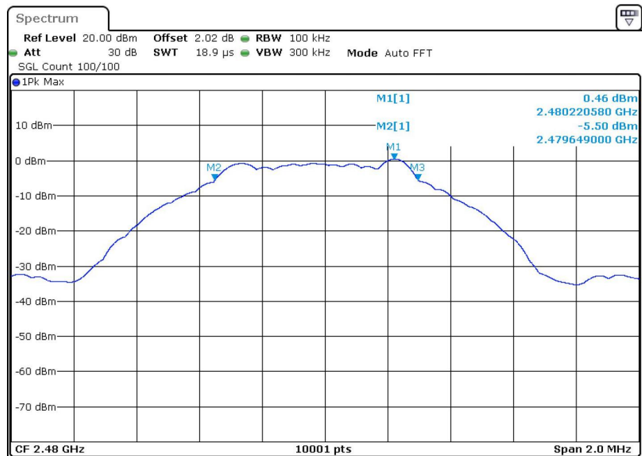
-6dB Bandwidth BLE 1M 2480MHz
