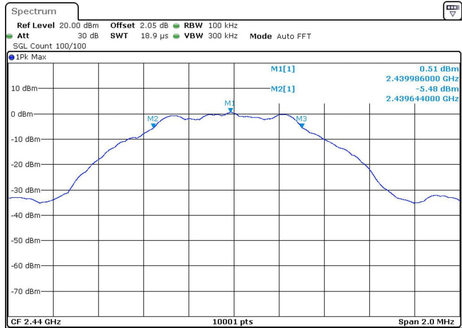
-6dB Bandwidth BLE 1M 2440MHz
