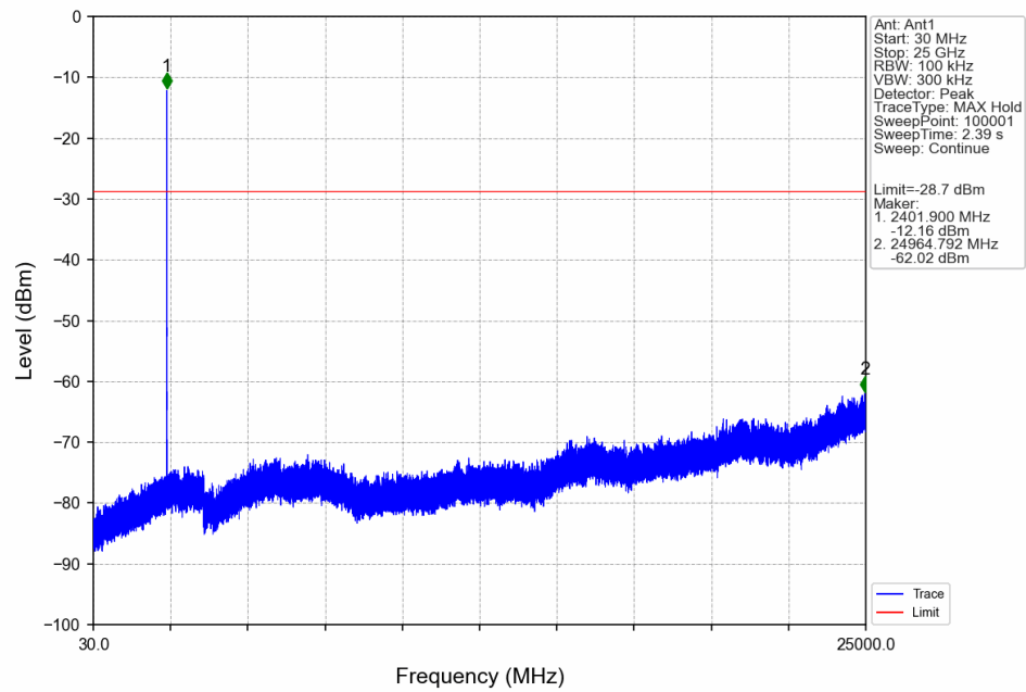
2.4G SRD_LCH_2403MHz_Ant1_NTNV
