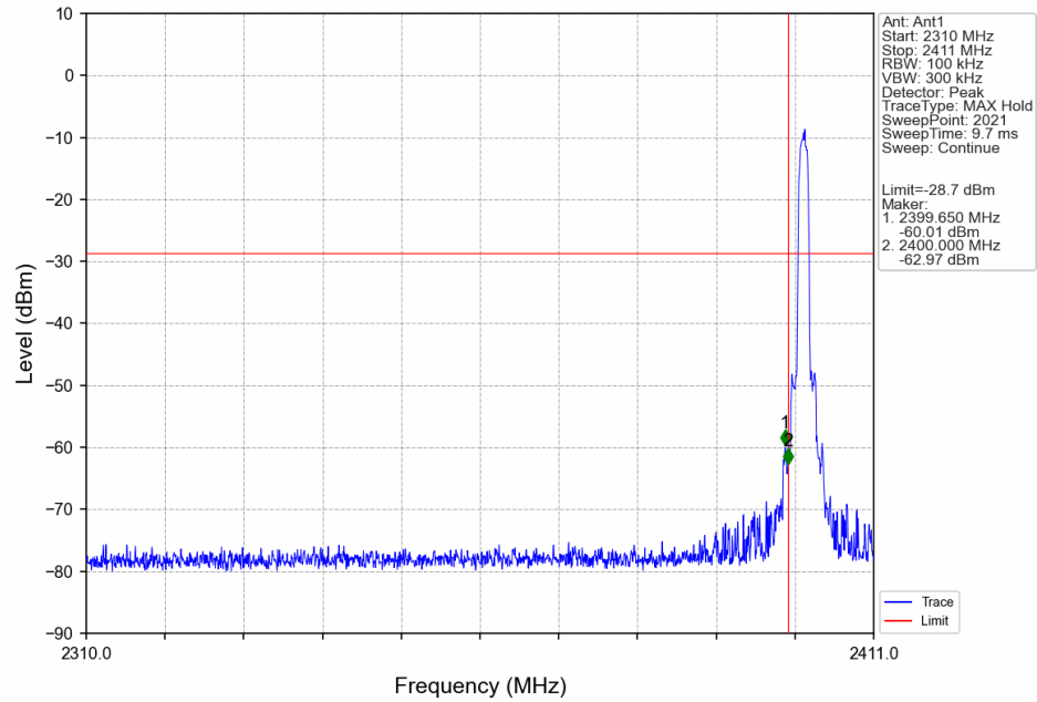
2.4G SRD_LCH_2403MHz_Ant1_NTNV
