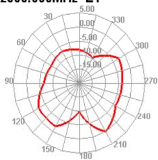
2500.000MHz E1
