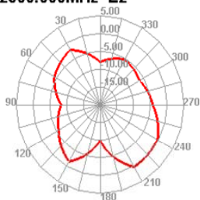
2500.000MHz E2
