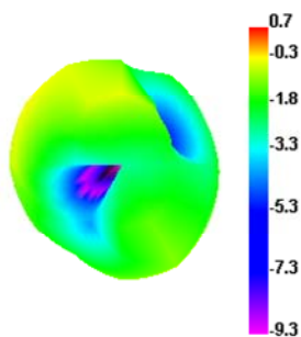
2500.000MHz E1
