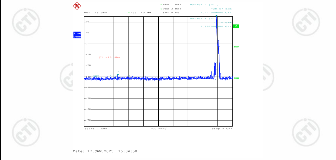
Band2-20MHz-QPSK-19100-1RB#0-Range2:1000~2000MHz
