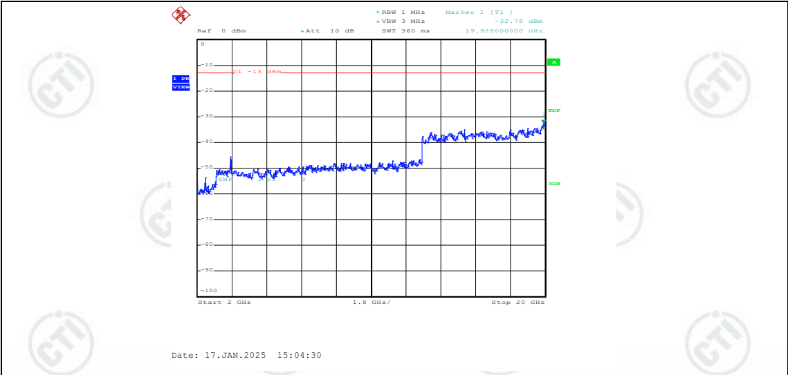
Band2-20MHz-QPSK-18900-1RB#0-Range3:2000~20000MHz
