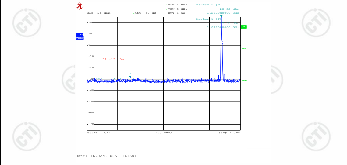
Band2-10MHz-QPSK-18900-1RB#0-Range2:1000~2000MHz
