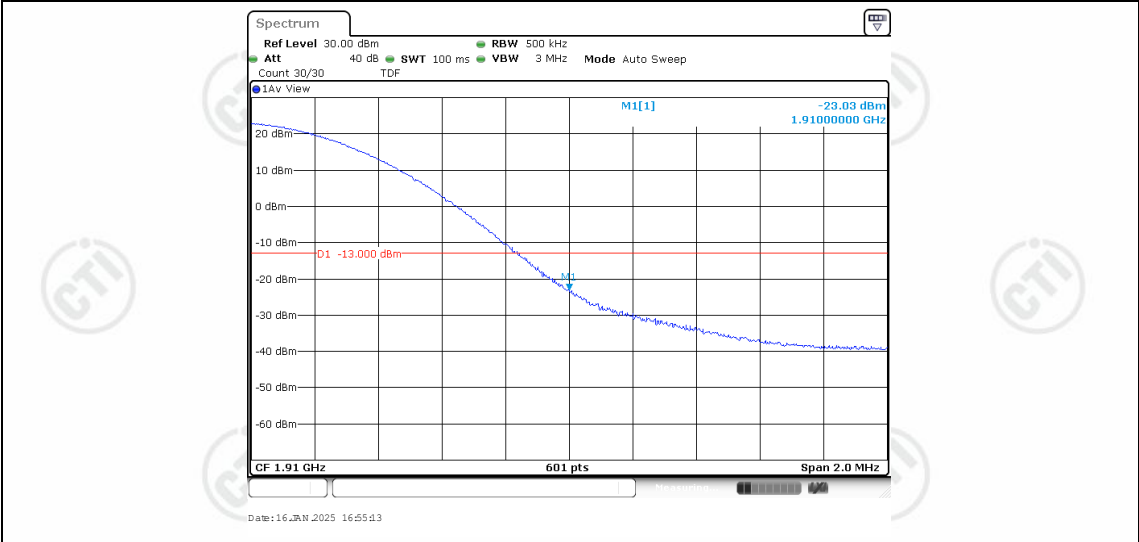
Band2-20MHz-QPSK-19100-1RB#99
