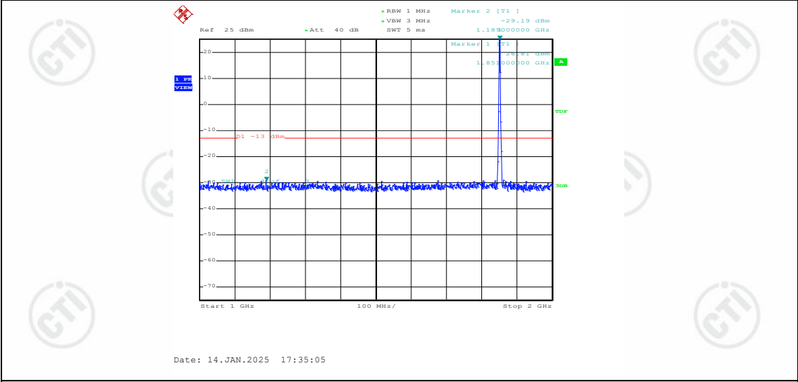
Band2-3MHz-QPSK-18615-1RB#0-Range2:1000~2000MHz
