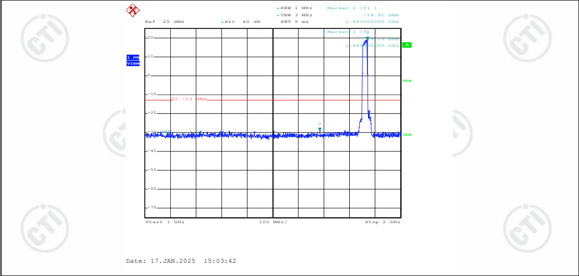
Band2-20MHz-QPSK-18700-1RB#0-Range2:1000~2000MHz
